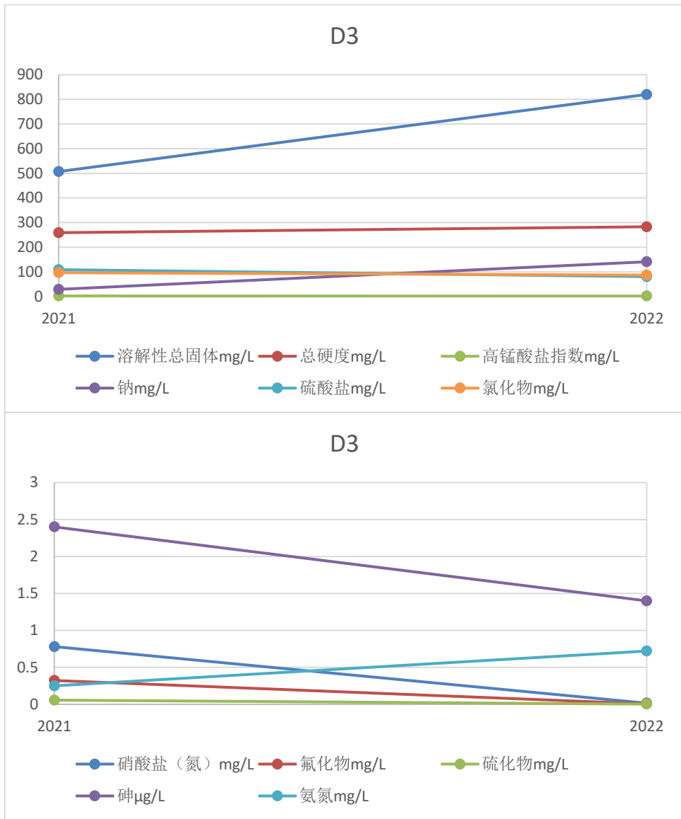
图8-2 D3点位污染物浓度变化趋势
